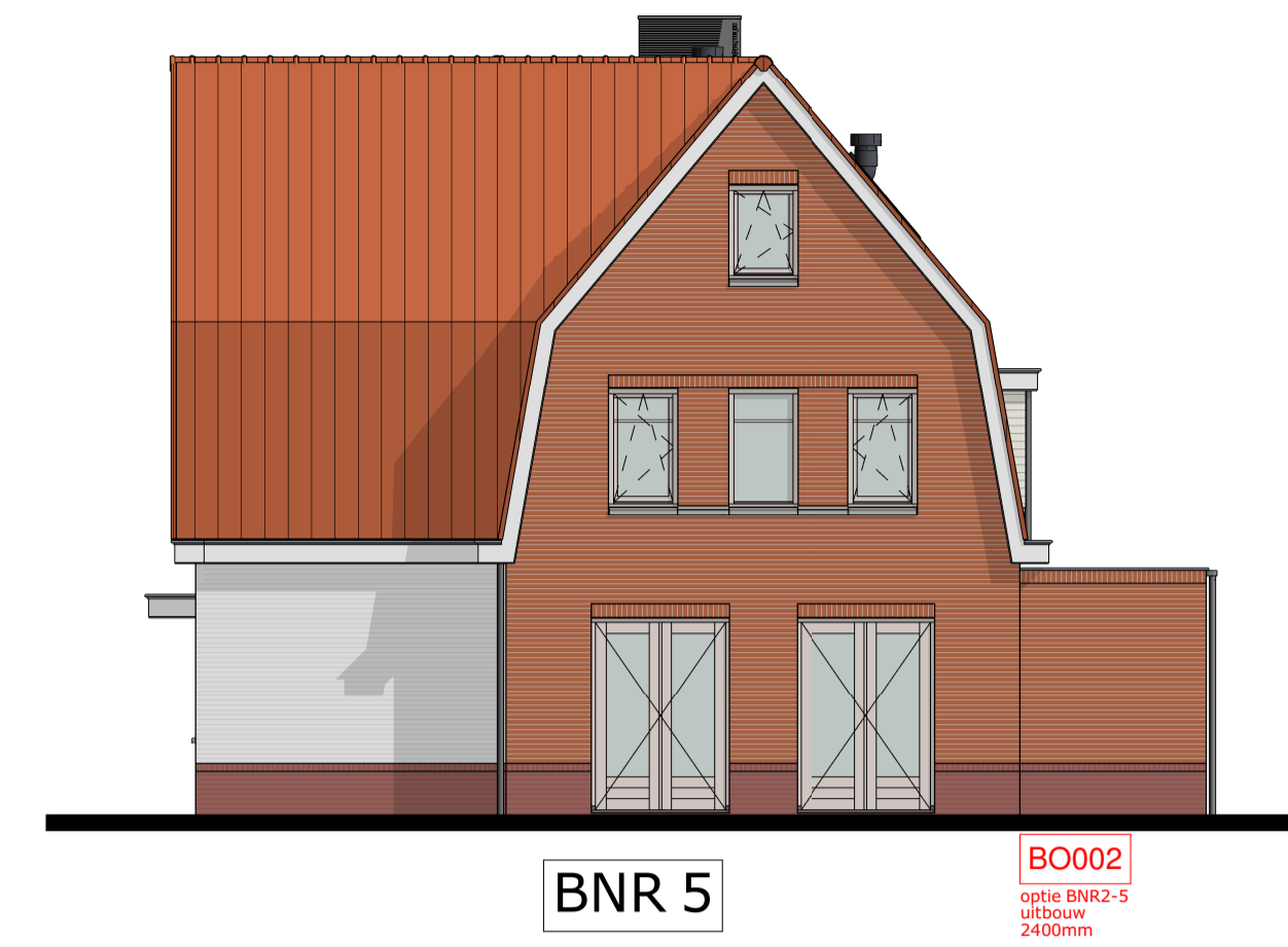
rechter zijgevel
