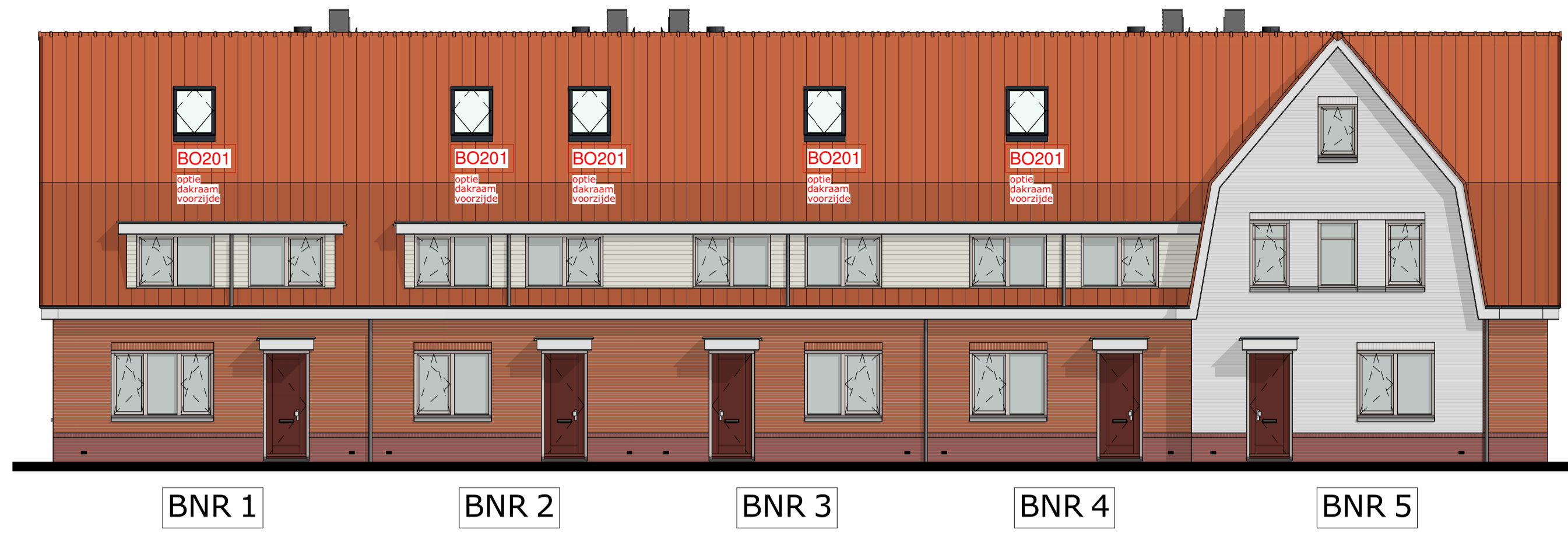
voorgevel
