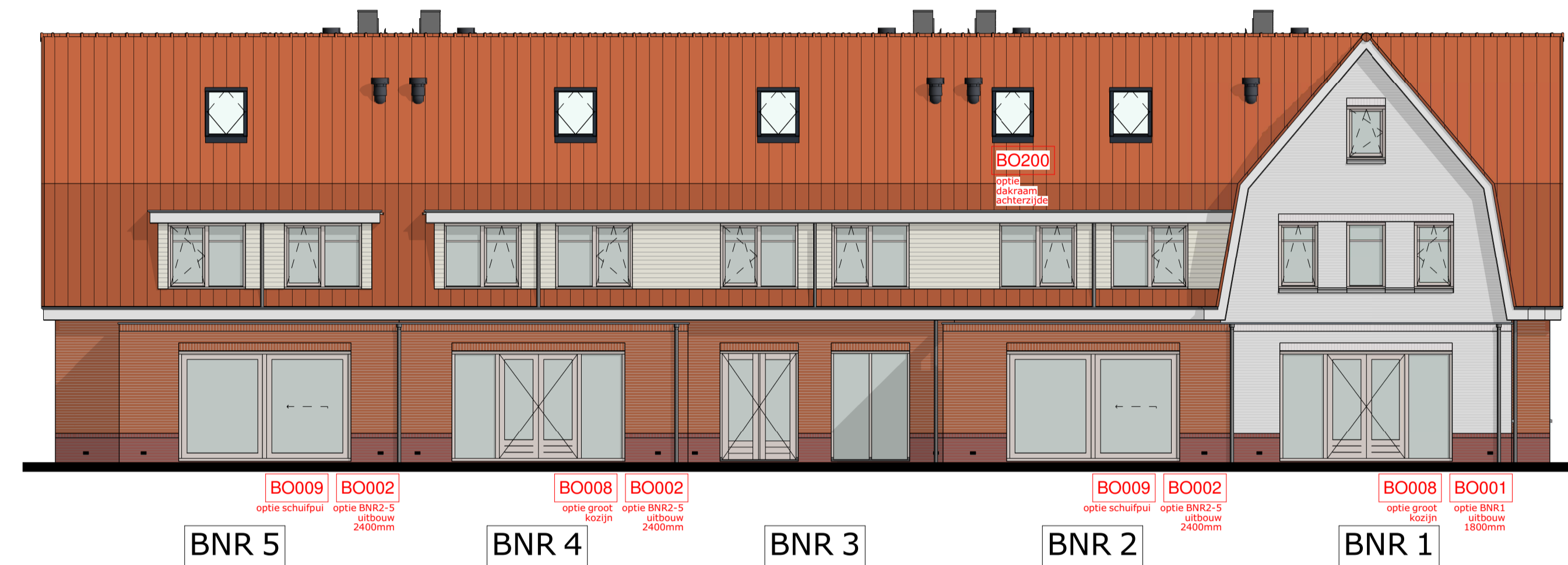
achtergevel
