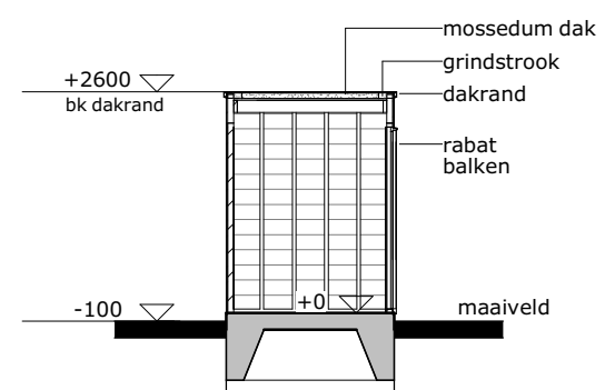
doorsnede B
