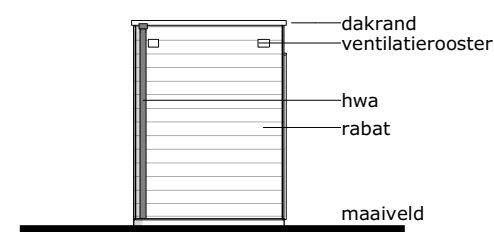
voorgevel
