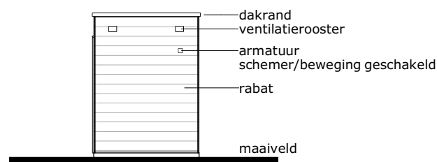
achtergevel
